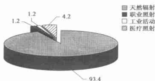
图 1 我国居民受电离辐射剂量份额
