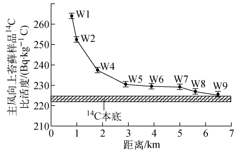
图 2 主风向上苔藓样品比活度随距离的变化
