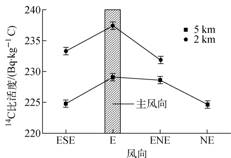
图3 不同半径上比活度与风向的关系
