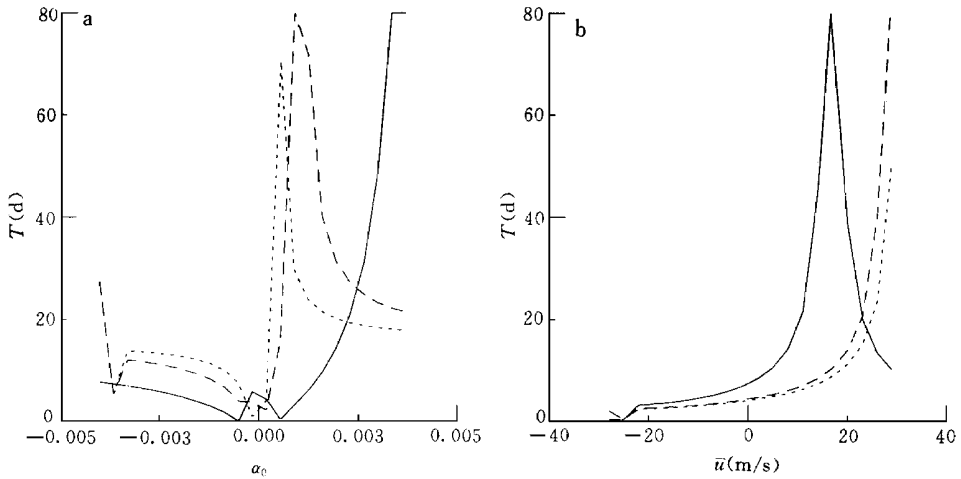
图 2 (a) T 随 \alpha_0 ( \bar{u} = 25 \text{ m/s} ) 和 (b) T 随 \bar{u} ( \alpha_0 = 0.002 ) 的变化 (实线: 曲线 1, 虚线: 曲线 2, 点线: 曲线 3 \alpha_0 = \partial v_s / \partial y , 均为取纬向 3 波时的波数 曲线 1, 2, 3 为 n = 0, 1, 2 的情况, 其它说明同图 1)
