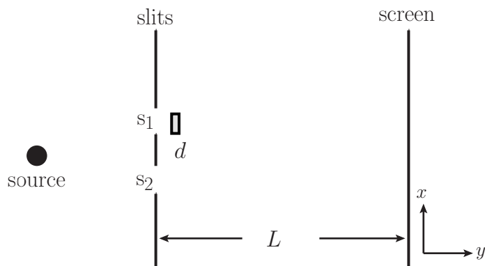
图 3.3: 测量对双缝干涉实验的影响
