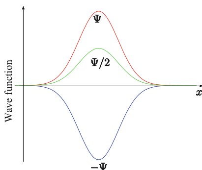
图 3.4: 等价的不同几率波函数
