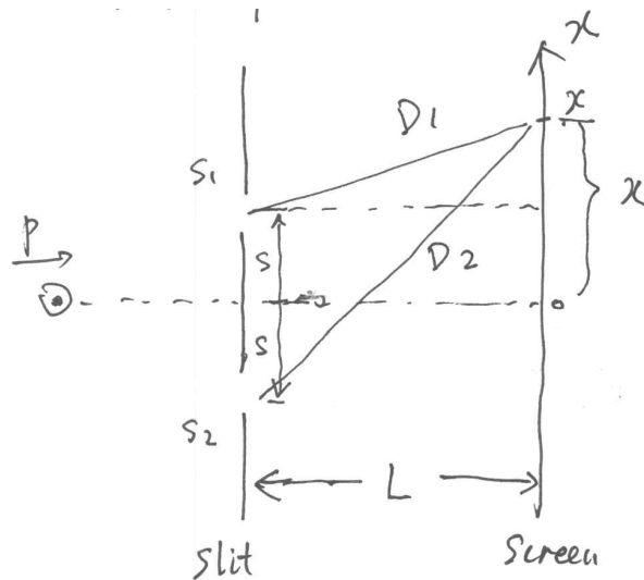
图 3.2: 双缝干涉实验
