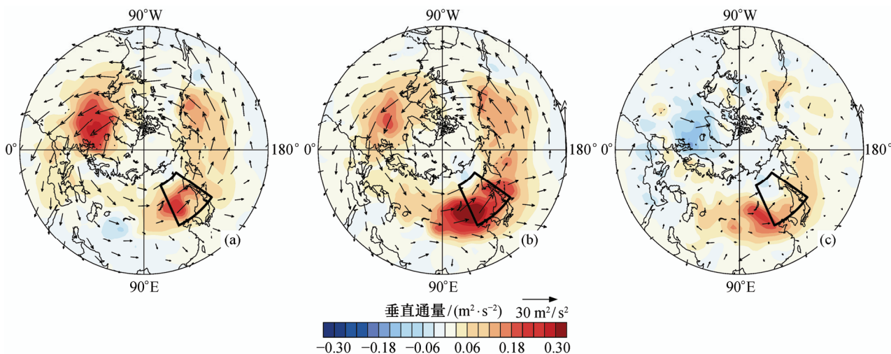
(a) NAM 正位相异常期间的 E-P 通量; (b) NAM 负位相异常期间的 E-P 通量; (c) NAM 负位相异常 E-P 通量减去 NAM 正位相异常 E-P 通量。黑色方框为东北冷涡的活动区域
