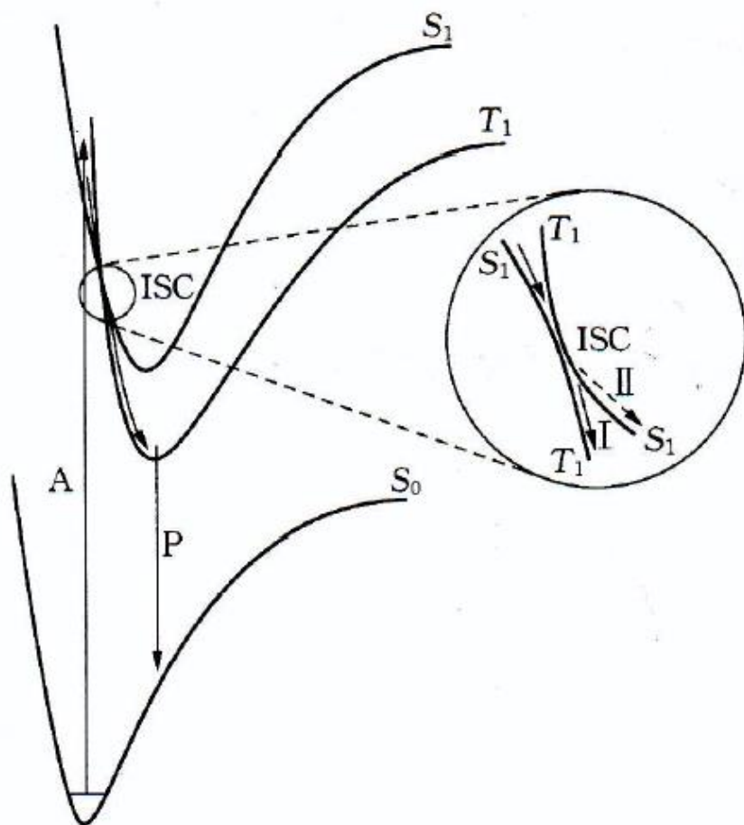
图 2.1.8 系间窜越 (ISC) 与磷光发射 (P)
